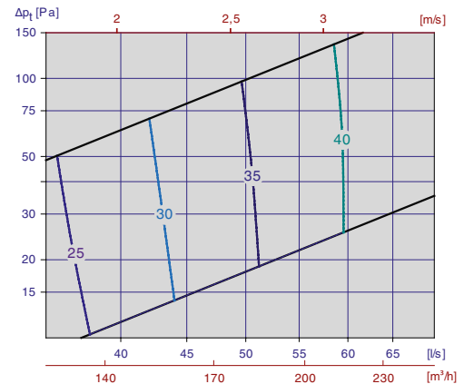
Diagram 6, Tilluft Orion-LØV m/Luna 160-160
