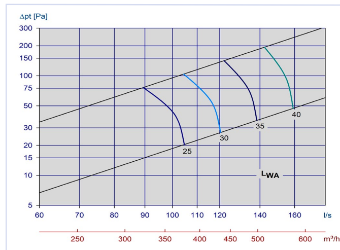
Diagram 29, Avtrekk Orion-LØV m/Luna 250-250
