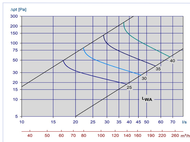
Diagram 19, Avtrekk Orion-LØV m/Luna 100-160
