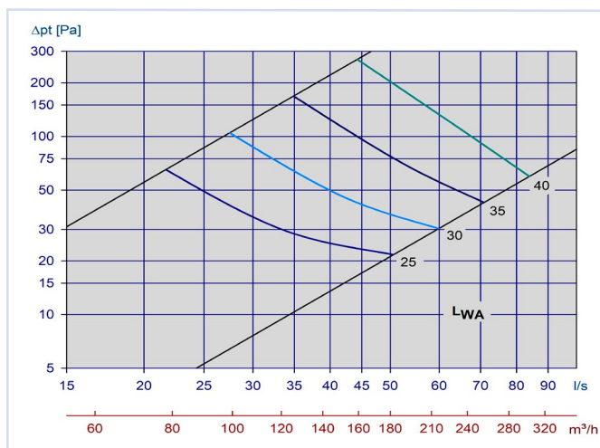
Diagram 21, Avtrekk Orion-LØV m/Luna 125-160
