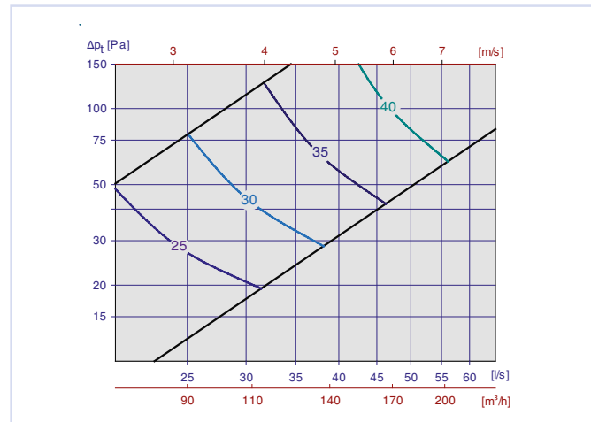
Diagram 2, Tilluft Orion-LØV m/Luna 100-160
