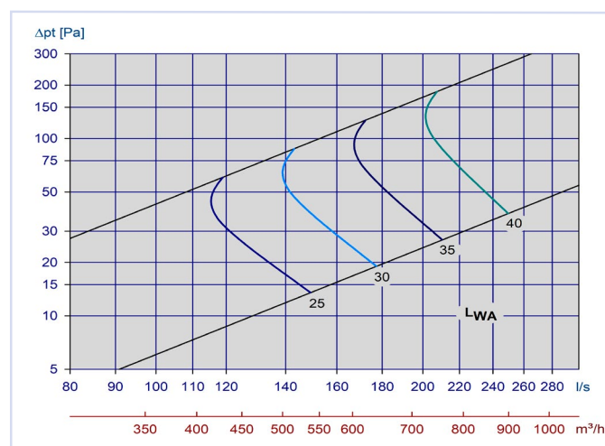
Diagram 31, Avtrekk Orion-LØV m/Luna 250-400
