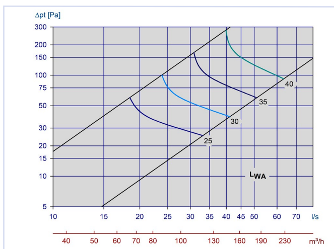
Diagram 18, Avtrekk Orion-LØV m/Luna 100-125
