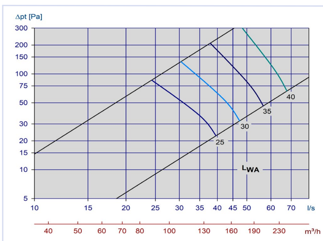
Diagram 20, Avtrekk Orion-LØV m/Luna 125-125
