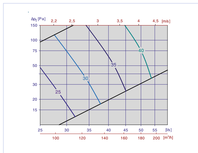
Diagram 4, Tilluft Orion-LØV m/Luna 125-160
