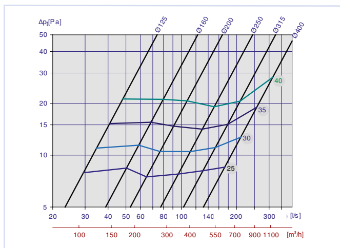
Diagram 17, Kapasitetsdiagram for Orion-LØV i kanalede
