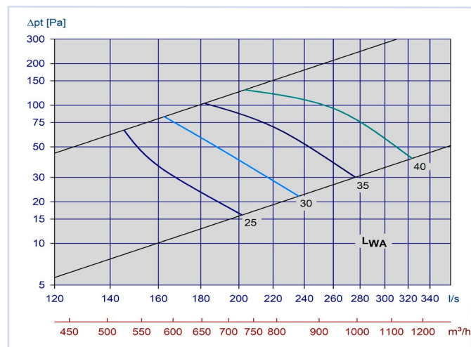
Diagram 33, Avtrekk Orion-LØV m/Luna 315-400
