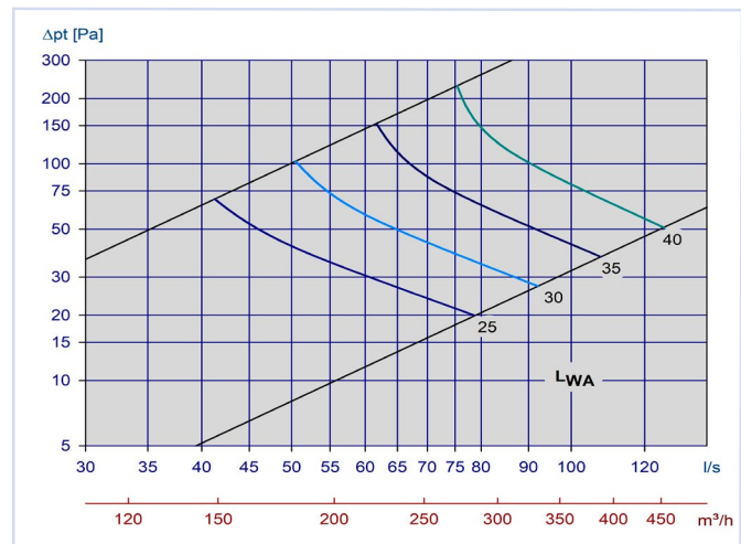
Diagram 25, Avtrekk Orion-LØV m/Luna 160-250
