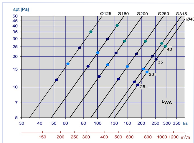
Diagram 34, Orion-LØV i kanalende, avtrekk
