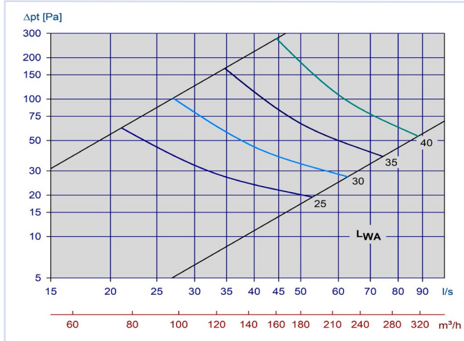
Diagram 22, Avtrekk Orion-LØV m/Luna 125-200
