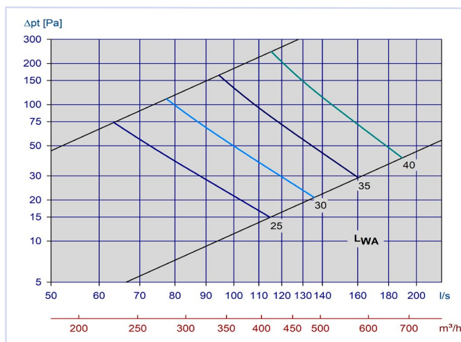
Diagram 28, Avtrekk Orion-LØV m/Luna 200-315
