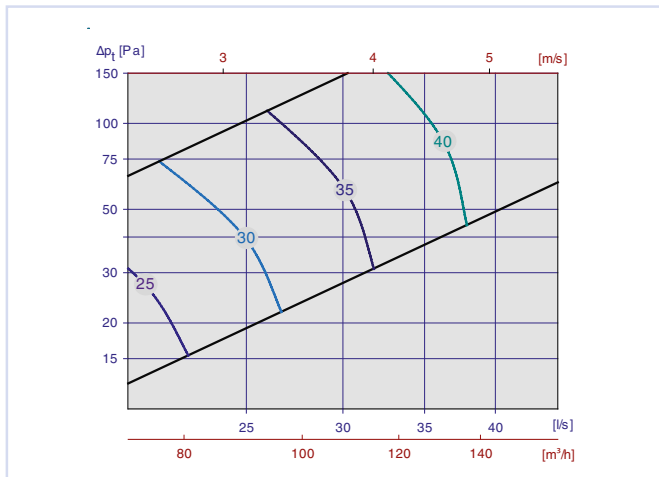
Diagram 1, Tilluft Orion-LØV m/Luna 100-125
