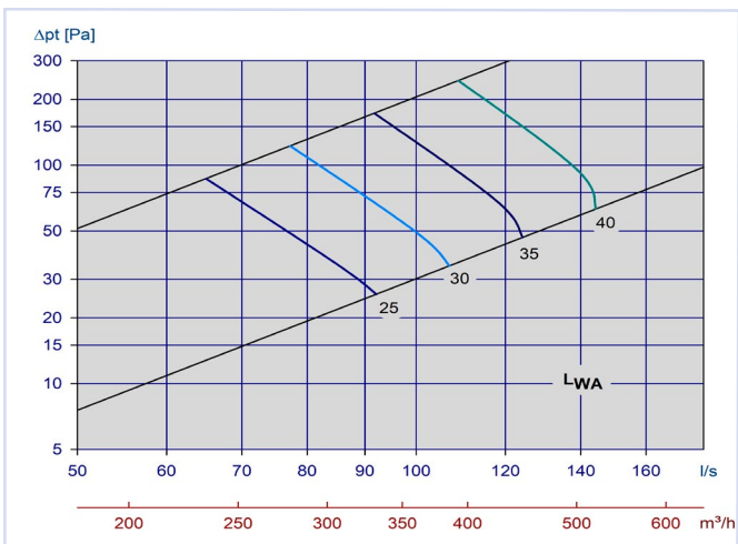
Diagram 26, Avtrekk Orion-LØV m/Luna 200-200
