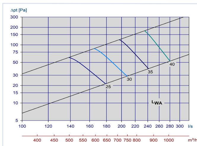
Diagram 32, Avtrekk Orion-LØV m/Luna 315-315
