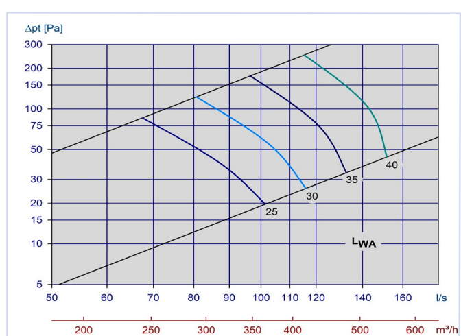
Diagram 27, Avtrekk Orion-LØV m/Luna 200-250
