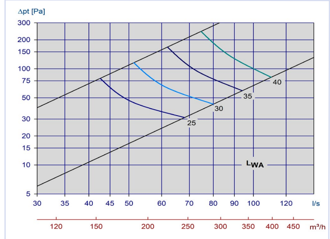
Diagram 23, Avtrekk Orion-LØV m/Luna 160-160
