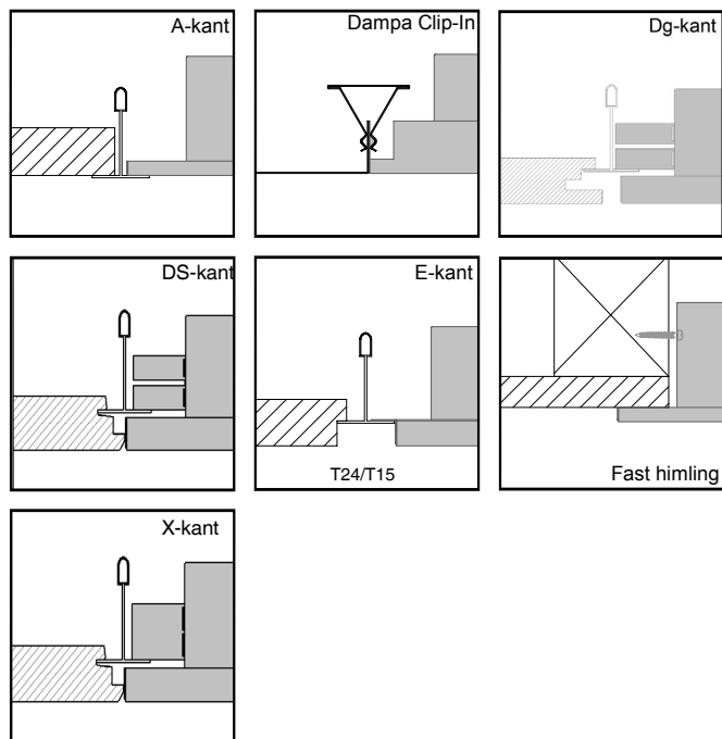
Figur 6, montasje
