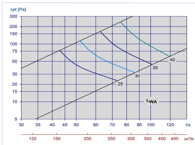
Diagram 24, Avtrekk Orion-LØV m/Luna 160-200
