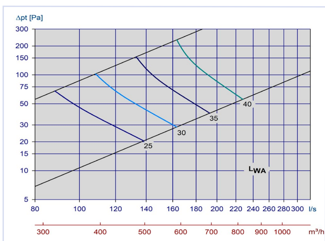
Diagram 30, Avtrekk Orion-LØV m/Luna 250-315
