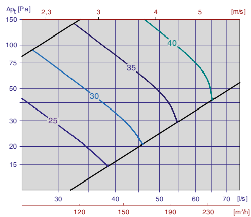
Diagram 5, Tilluft Orion-LØV m/Luna 125-200
