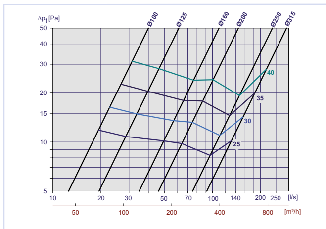
Diagram 16, Tilluft kapasitetsdiagram for LØV-R i kanalende.
