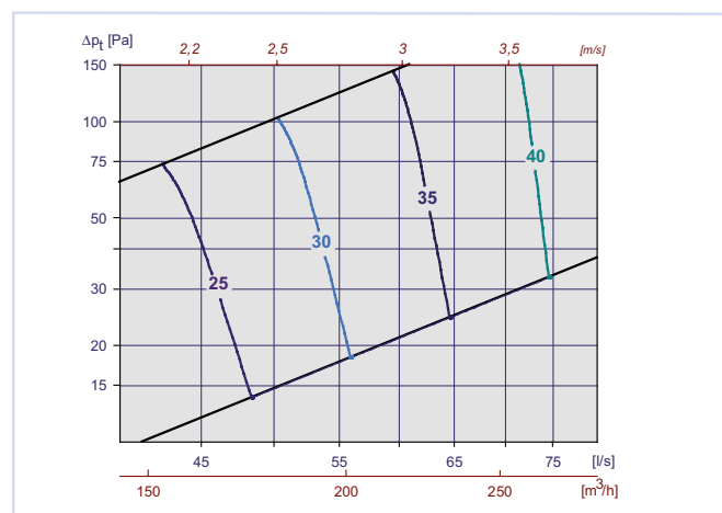
Diagram 8, Tilluft LØV-R m/Luna 160-200
