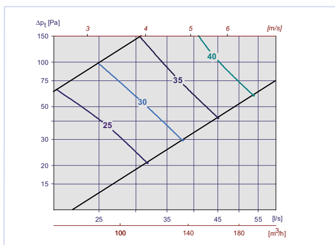
Diagram 3, Tilluft LØV-R m/Luna 100-160
