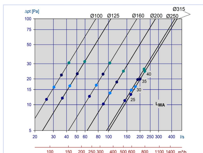
Diagram 33, LØV-R i kanalede
