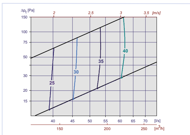
Diagram 7, Tilluft LØV-R m/Luna 160-160
